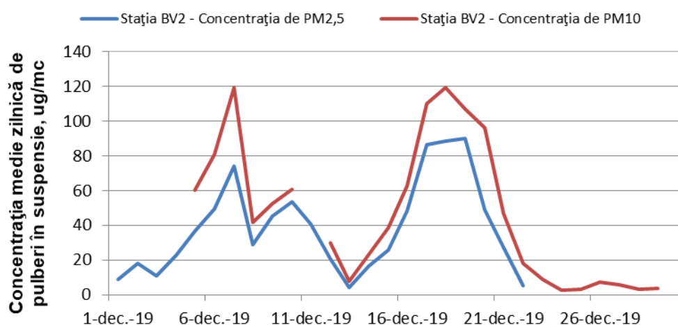
Figura 1.1.2.4.4 Evoluția mediilor zilnice de PM 2,5 și PM 10 în luna decembrie
