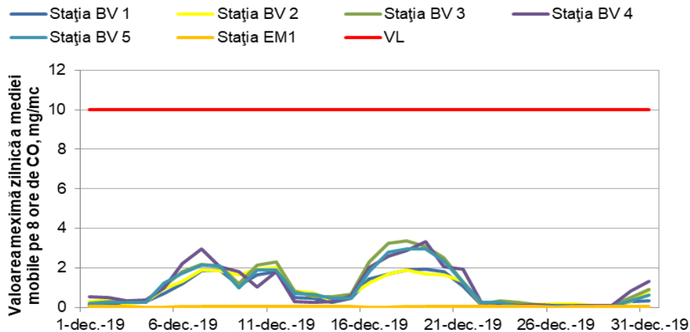
Figura 1.1.2.5.1. Evoluția maximelor zilnice ale mediei mobile de CO în luna decembrie
