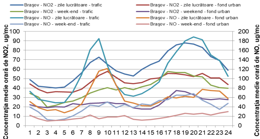
Figura 1.1.2.2.3. Ciclu zilnic al oxizilor de azot în timpul săptămânii
