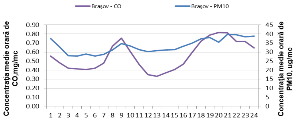
Figura 1.1.2.4.3: Ciclul zilnic al PM10 și CO în Brașov
