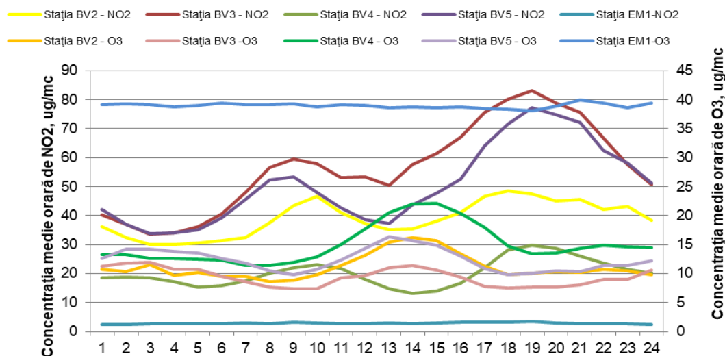
Figura 1.1.2.3.3. Ciclul zilnic al O 3 și NO 2
