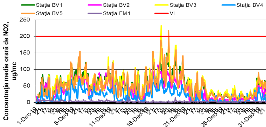
Figura 1.1.2.2.1. Evoluția mediilor orare de NO 2 în luna decembrie
