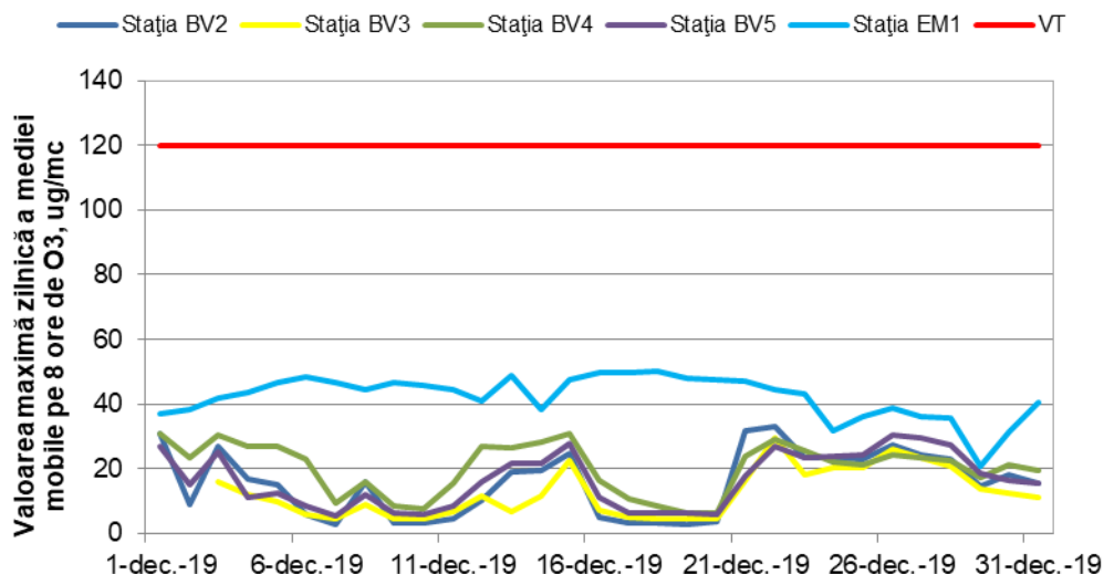
Figura 1.1.2.3.1. Evoluția maximelor zilnice ale mediilor mobile pe 8 ore de O 3 în luna decembrie
