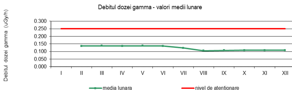
Fig. 1.3.3. Debitul dozei gamma în aer
