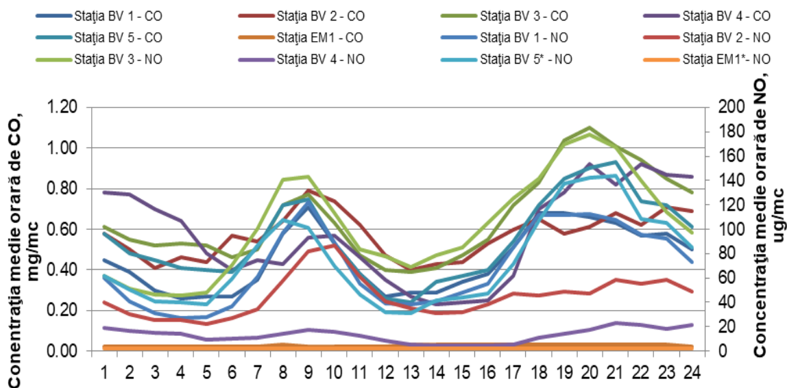
Figura 1.1.2.2.4. Ciclu zilnic al NO și CO
