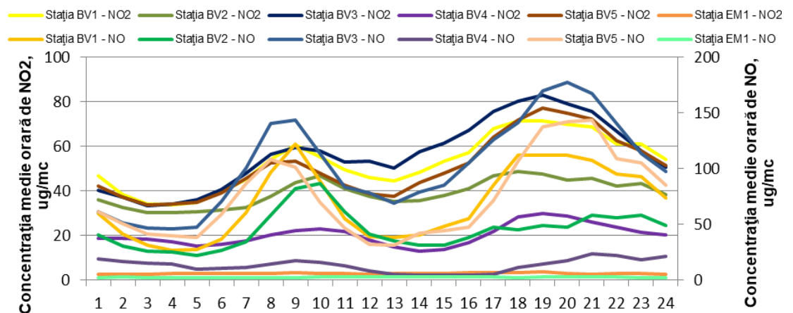
Figura 1.1.2.2.2. Ciclul zilnic al NO 2 și NO
