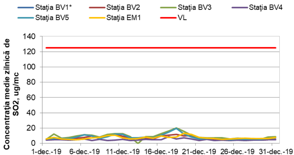
Figura 1.1.2.1.1. Evoluția mediilor zilnice de \text{SO}_2 în luna decembrie
